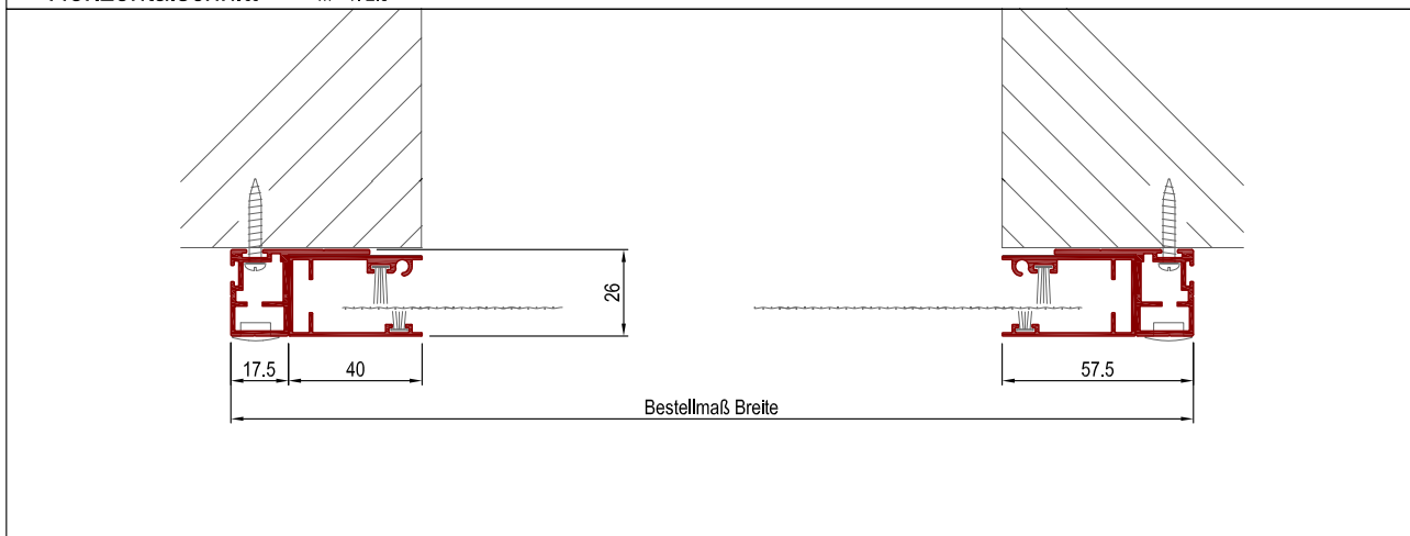
Horizontalschnitt
