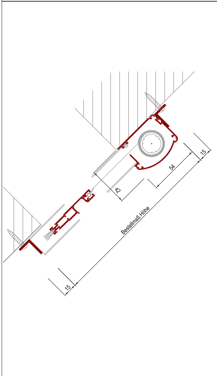
Vertikalschnitt
