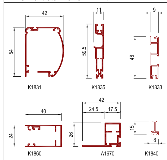
Verwendete Profile
