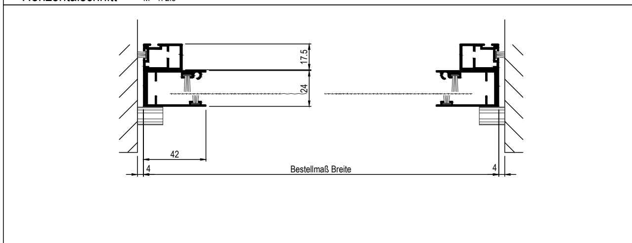
Horizontalschnitt
