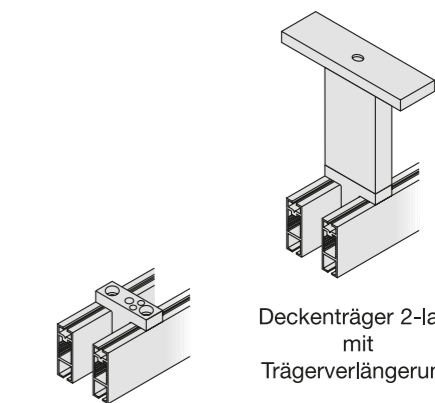
Deckenträger 2-lauf
