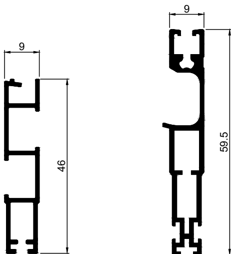
Art.Nr. K1833 Bezeichnung Rollo Zugschiene
