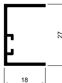
Art.Nr. K1880 Bezeichnung Türrollo-Verschlusschiene
