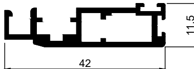
Art.Nr. A1130 Bezeichnung Spannrahmenprofil Typ I mit Bürstenführung
