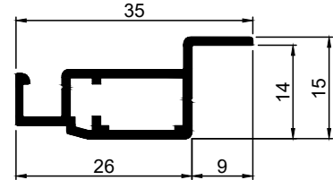
Art.Nr. A1019 Bezeichnung Spannrahmenprofil mit abgesetztem Falz
