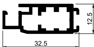
Art.Nr. A1240 Bezeichnung Drehrahmenprofil für Duplertextüre
