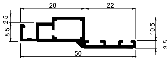
Art.Nr. A2020 Bezeichnung Spannrahmenprofil Typ II mit Falz 22 mm, Bürsten- und Schlittenführung
