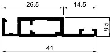
Art.Nr. A2014 Bezeichnung Spannrahmenprofil Typ II mit Falz 14,5 mm und Bürstenführung
