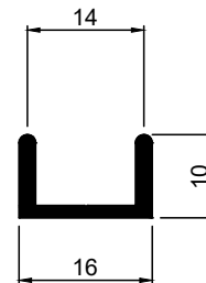
Art.Nr. A1360 Bezeichnung U - Profil Führungsschiene für Schiebetüre
