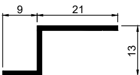
Art.Nr. A7060 Bezeichnung Z - Profil Befestigungsschiene für Spannrahmen
