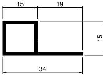
Art.Nr. A1570 Bezeichnung Einbaurahmenprofil
