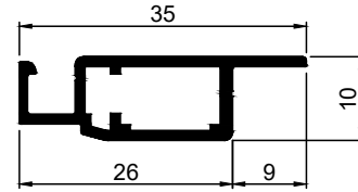
Art.Nr. A1012 Bezeichnung Spannrahmenprofil mit Falz 9 mm
