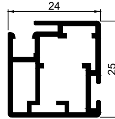
Art.Nr. A1580 Bezeichnung Einbaurahmenprofil groß
