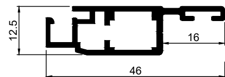
Art.Nr. A1230 Bezeichnung Drehrahmenprofil mit Falz innen
