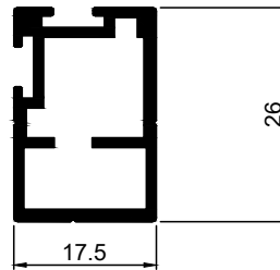
Art.Nr. A1690 Bezeichnung Einbaurahmenprofil Multi
