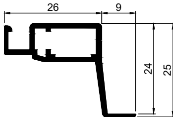
Art.Nr. A1024 Bezeichnung Spannrahmenprofil mit abgesetztem Falz 24
