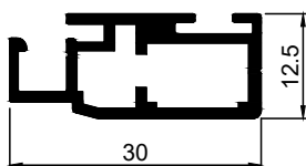
Art.Nr. A1210 Bezeichnung Drehrahmenprofil
