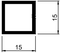
Art.Nr. A1515 Bezeichnung RR - Hohlpr.- Einbaur. 15x15x1.2
