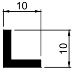
Art.Nr. A8110 Bezeichnung L - Winkelprofil 10x10x2
