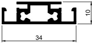
Art.Nr. A1250 Bezeichnung Sprossenprofil gewebeiteilend
